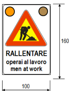
Figura 18: pannello composito di presegnalazione per lavori eseguiti lungo le corsie di decelerazione o sulle rampe di svincolo, dotato di 2 lampade a led ad alta efficienza diam. 200 mm. Superficie della targa non inferiore a 1,5 mq con lato del triangolo lavori in corso non inferiore a 90 cm. Posizionamento sul margine destro in coincidenza dell’ago di inizio della decelerazione e ripetuto in condizioni di non perfetta visibilità.
